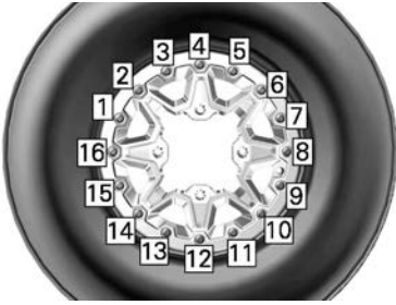
TYPBILD - SLUTLIG ÅTDRAGNINGSEKVENSENS
