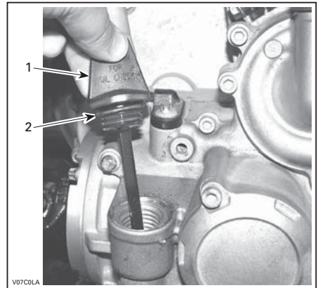
LADO DIREITO DO MOTOR
