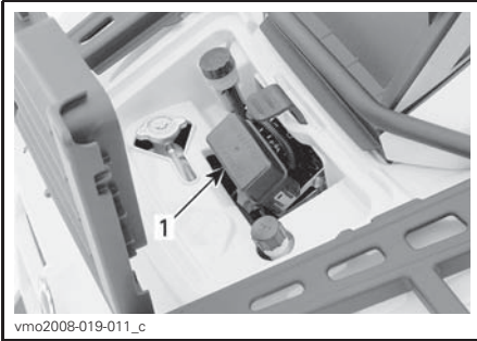
1. Caixa de fusíveis dianteira
