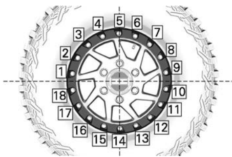
典型示例 - 最终紧固顺序
