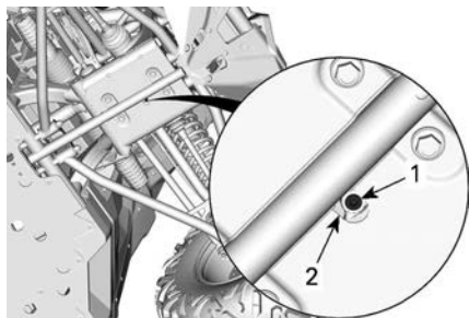
车辆底部
