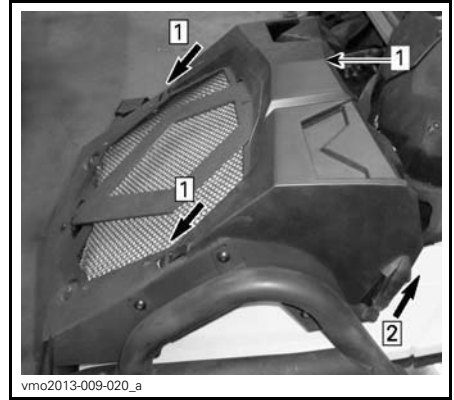
Étape 1: Déverrouiller les loquets Étape 2: Appuyer sur les pattes
