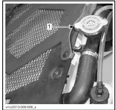
1. Bouchon du radiateur
