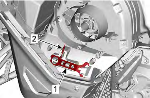
典型 - 驱动皮带护罩工具位置
