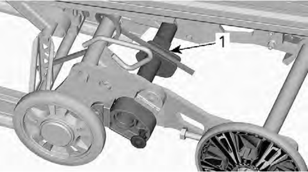
1. Esijännityksen säätönokka
