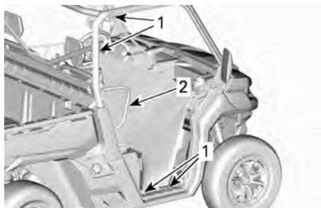
1. Locaties waar het zijnet wordt aangespannen 2. Schouderbescherming
