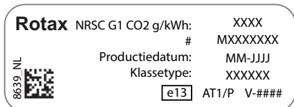
TYPISCH - NRMM-IDENTIFICATIELABEL
