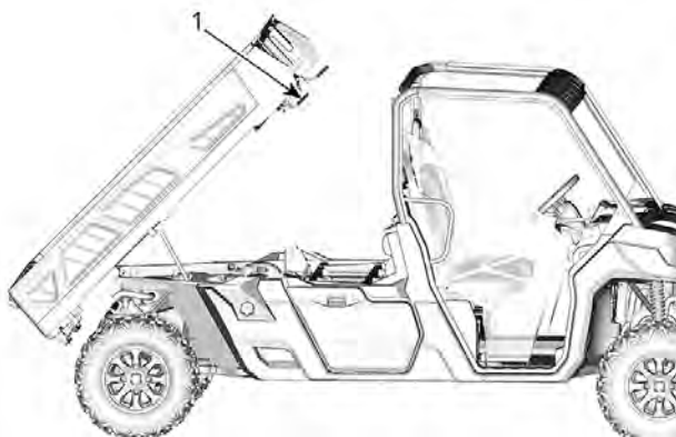
1. Ontgrendelingshendels
