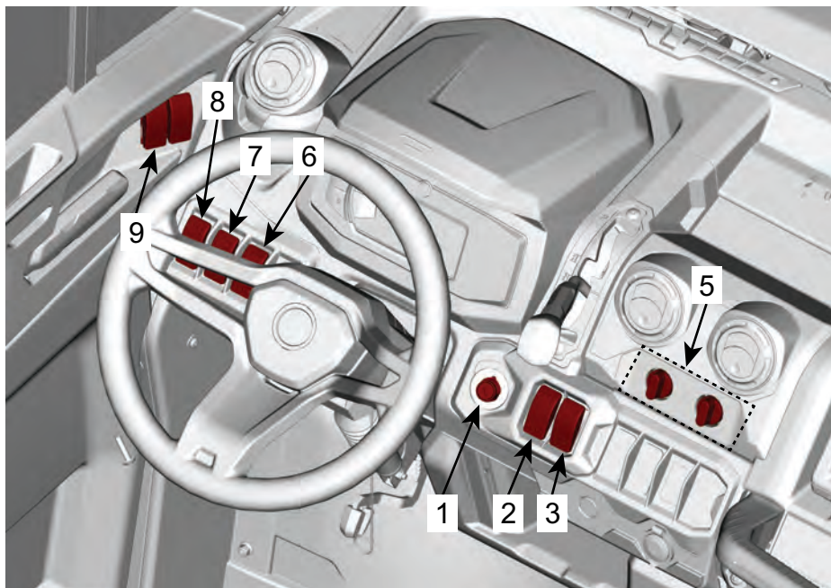
CONFIGURAZIONE TIPICA - MODELLO CON ABITACOLO CON SISTEMA DI RISCALDAMENTO IN FIGURA
