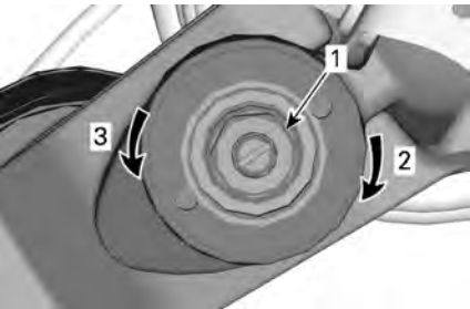
高速压缩阻尼 (使用 17 MM 螺丝刀)
