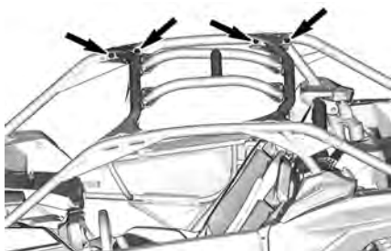
HÖGER SIDOBUR
