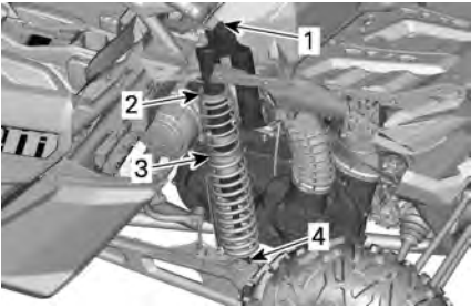
SITUAZIONE TIPICA - CON SMORZAMENTO IN ESTENSIONE - SOSPENSIONE POSTERIORE
