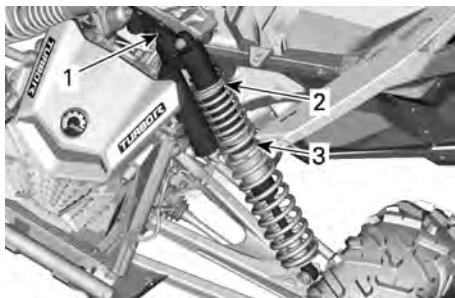
TÍPICO - SEM AMORTECIMENTO DO REBOTE - SUSPENSÃO DIANTEIRA
