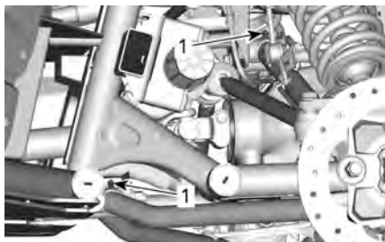
TÍPICO - SUSPENSÃO DIANTEIRA
