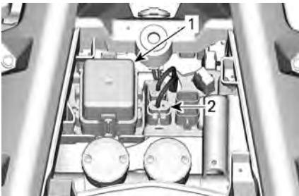
1. Caixa de fusíveis dianteira 2. Fusível da DPS
