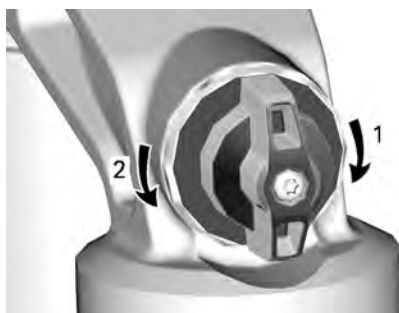
TÍPICO - AJUSTE DE LA SUPERPOSICIÓN - AMORTIGUADOR TRASERO
