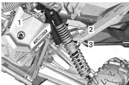
TYPIQUE - SANS AMORTISSEMENT DE REBOND - SUSPENSION AVANT
