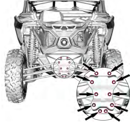
TYPIQUE - BARRE STABILISATRICE ARRIÈRE
