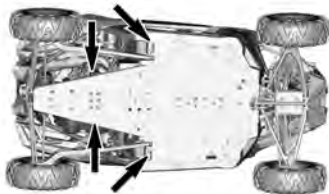
POSICÕES DE APOIO DO MACACO - PARTE TRASEIRA DO VEÍCULO
