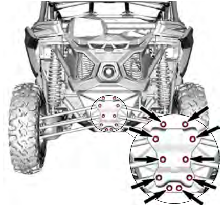
TÍPICO - BARRA ESTABILIZADORA TRASEIRA
