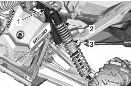
TÍPICO - SEM AMORTECIMENTO DO REBOTE - SUSPENSÃO DIANTEIRA
