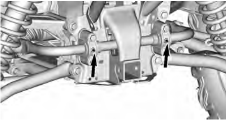
TIPIQUE - BARRE STABILISATRICE ARRIÈRE
