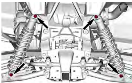
TIPIQUE — FIXATIONS D'AMORTISSEUR ARRIÈRE
