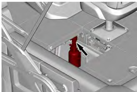
ACTIONNEUR CHARGÉ
