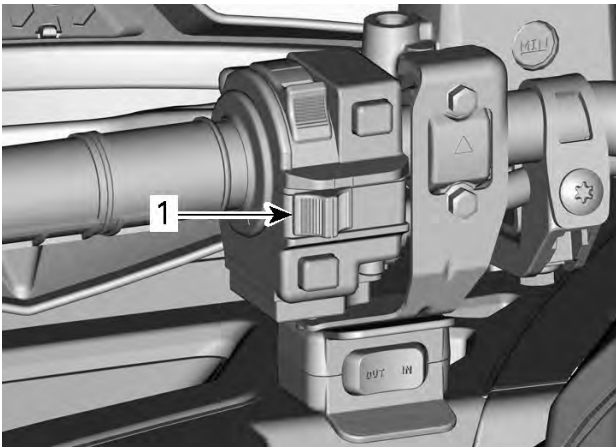
1. Motorns stoppreglage
