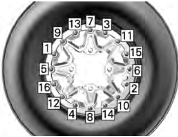
TIPIQUE - SÉQUENCE DE SERRAGE
