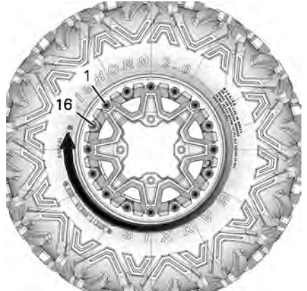
TIPIQUE - SÉQUENCE DE SERRAGE FINAL
