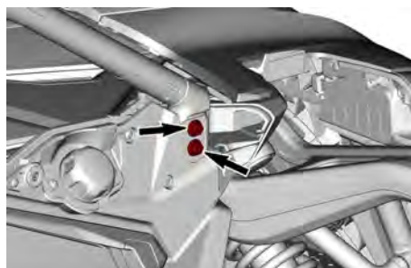
FIXATIONS AVANT — TYPIQUE
