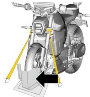
Framhjulslås
