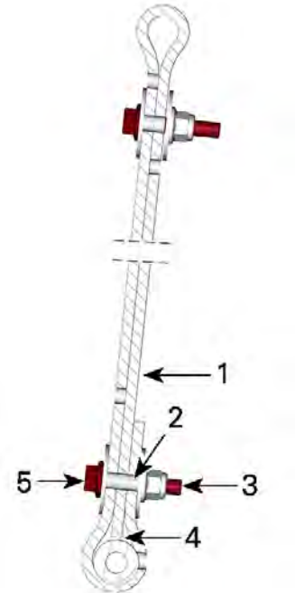
可调式止动带长端长度设置 ( 第 1 个孔 , 出厂设置 )
