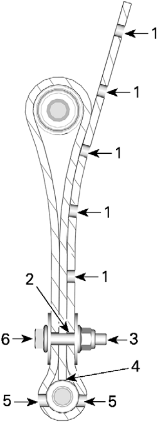
止动带位置 6 ( 第 6 个孔 ) 1. 自由孔 2. 从端部算起的第 6 个孔 3. 朝后 4. 接触止动带轴的止动带端部 5. 螺钉头和螺帽之间的两个孔开口 6. 朝前
