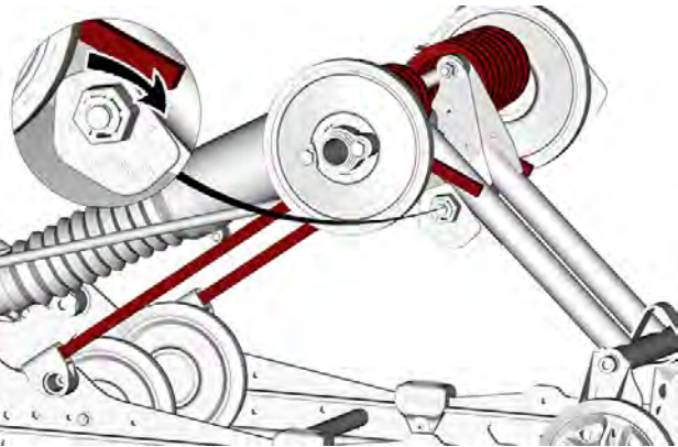
左侧弹簧预载调节 - 典型示例
