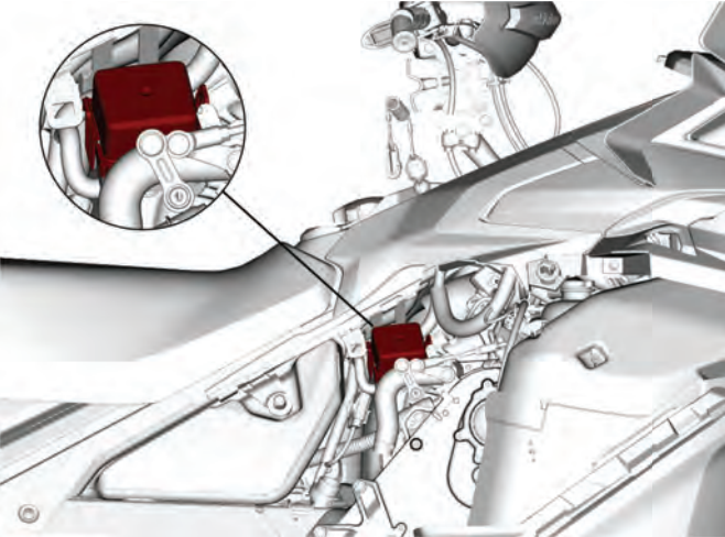
典型示例 - 保险丝盒 1 (FB1)
