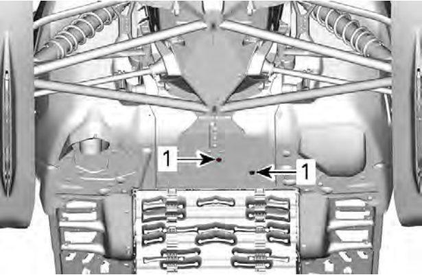
1. 固定螺钉
