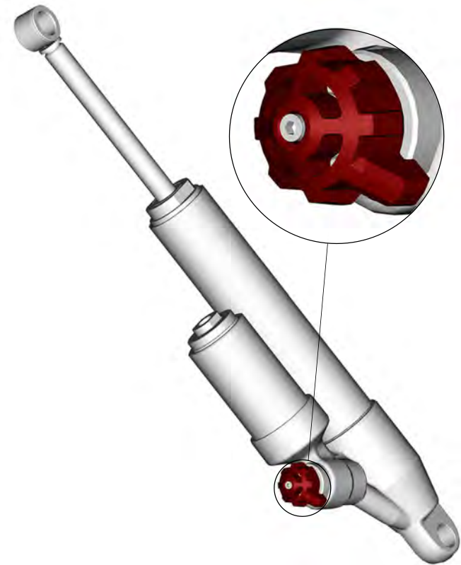
3 点式压缩阻尼调节旋钮
