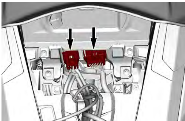
4. 拆下两颗固定上部车身模块支架的螺钉。
