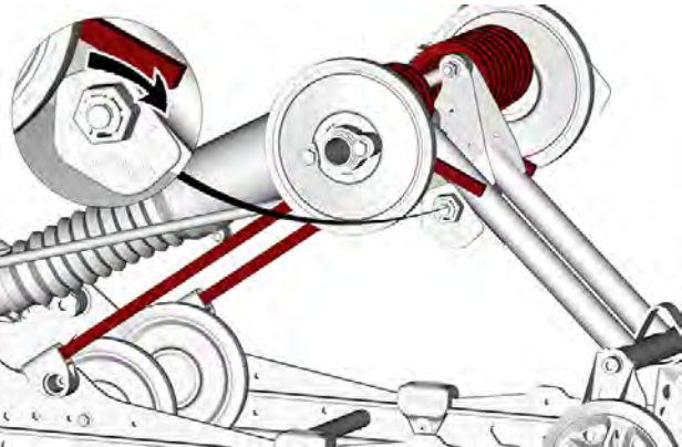
左侧弹簧预载调节 - 典型示例
