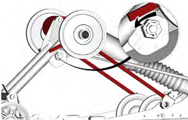
右侧弹簧预载调节 - 典型示例
