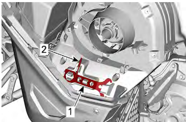
代表例 - ドライブベルトガードツールの位置
