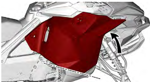
3. Kiinnitä sivupaneeli salvoilla.
