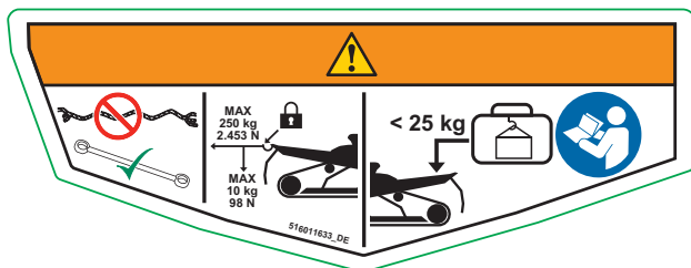
TRANSPORTBEREICH – WARNSCHILD
