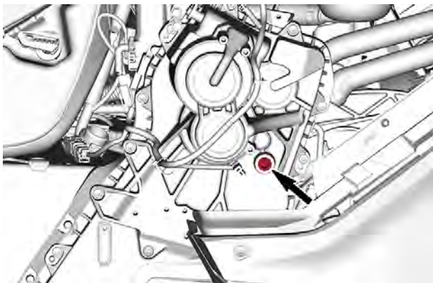
注油塞
