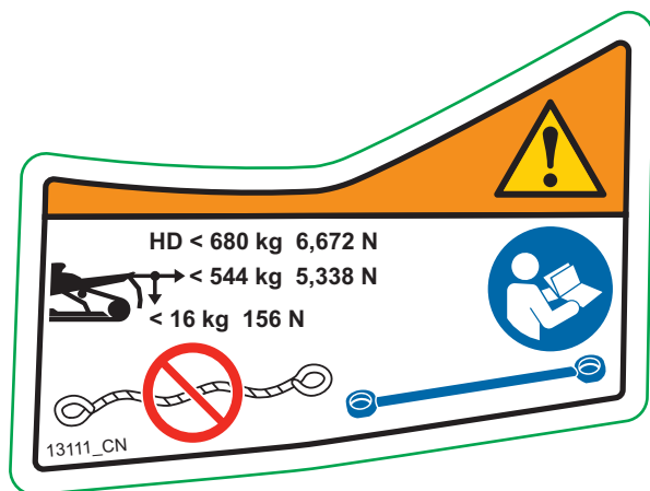
RANGER PRO 的牵引能力 - 警告标签
