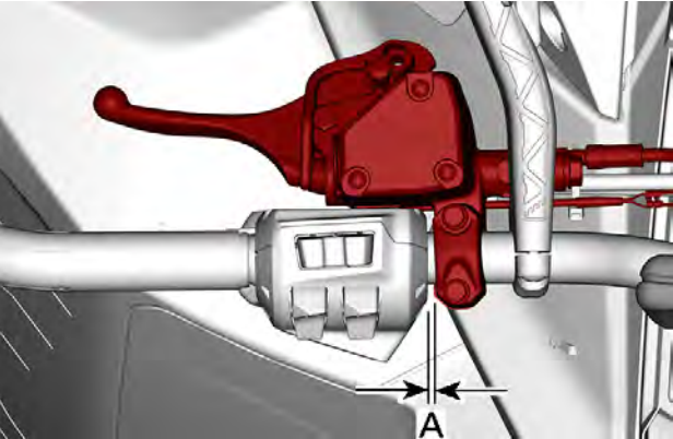
A. 多功能开关侧面与制动杆侧面之间应留出 0 至 15 mm 的距离
