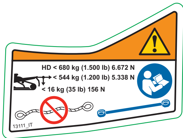
CAPACITÀ DI TRAINO RANGER PRO - ETICHETTA DI AVVERTENZA
