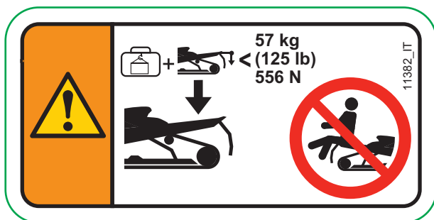
CAPACITÀ DI CARICO MASSIMA DI RANGER PRO - ETICHETTA DI AVVERTENZA
