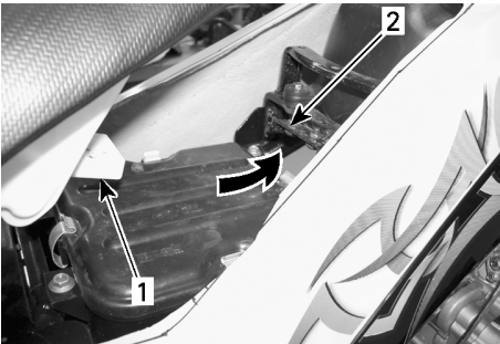
1. Tab 2. Hook
