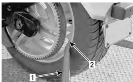
TÍPICO - SUJECIÓN DE LA RUEDA TRASERA
