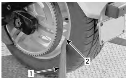
BAKHJULSFÖRANKRING – TYPBILD
