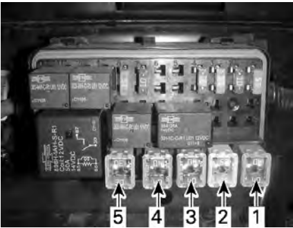
J-KASTEN-SICHERUNGEN – LINKER SICHERUNGSKASTEN
