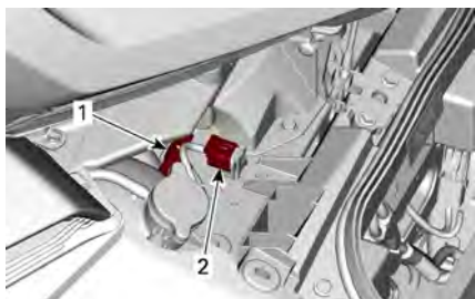
1. Diagnostisiliitin (BUDS2:ta varten)
