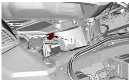
1. Connecteur de diagnostic (pour BUDS2)
