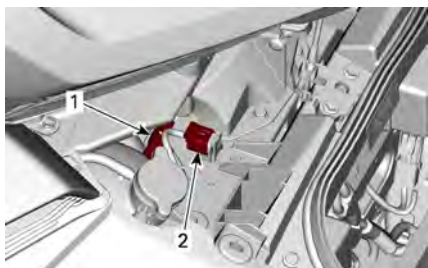
1. Connecteur de diagnostic (pour BUDS2) 2. Connecteur à 6 broches OBD2
