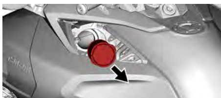
代表例 - エアインテークサイレンサーからの エアフィルターの取り外し
