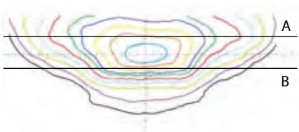
TYPISCH – SCHEINWERFERSTRAHL AUF DER TESTOBERFLÄCHE
