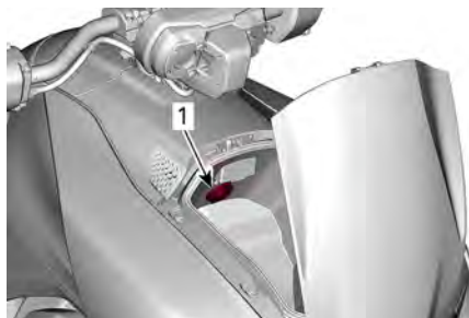
1. Conector USB doble
