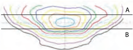
TÍPICO: REFLEJO DE FAROS EN LA SUPERFICIE DE PRUEBAS
