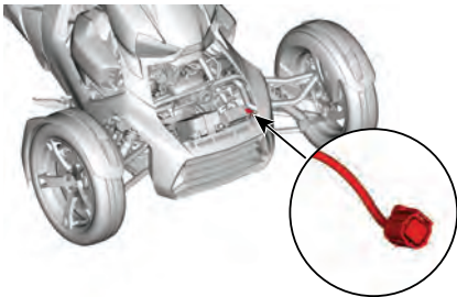
UBICACIÓN DEL CONECTOR DEL OBD
