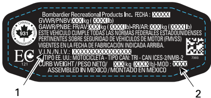
ETIQUETA DEL NÚMERO DE IDENTIFICACIÓN DEL VEHÍCULO
