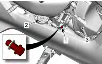
UBICACIÓN DEL TAPÓN DEL NIVEL DE ACEITE DE LA CAJA DE CAMBIOS
