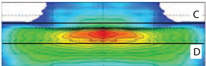
TÍPICO: REFLEJO DE FAROS EN LA SUPERFICIE DE PRUEBAS
