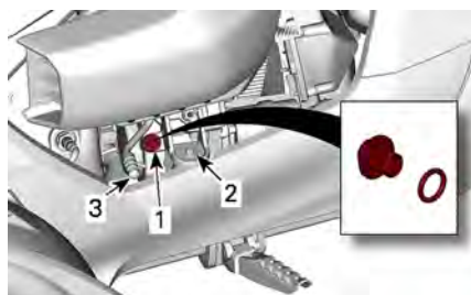
ギヤボックスオイルフィラープラグの位置
