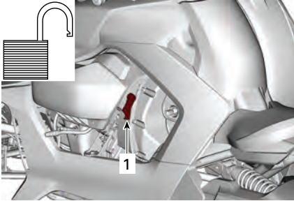
1. Parkeerhendel in ontgrendelde stand (uitgeschakeld)
