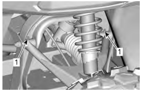
1. Puntos de engrase del brazo de la suspensión
