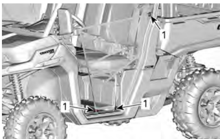
1. Ubicaciones de ajuste de las redes laterales
