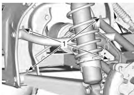
1. Graisseurs du bras de suspension arrière
