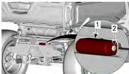
1. Cache de l'ampoule de la plaque d'immatriculation 2. Vis de fixation
