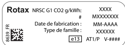
TYPIQUE - ÉTIQUETTE D'IDENTIFICATION NRMM
