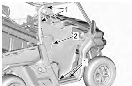
1. Posizione delle regolazioni per le protezioni laterali 2. Salvaspalla
