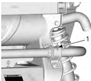
1. Punto di ingrassaggio della boccola della barra stabilizzatrice posteriore
