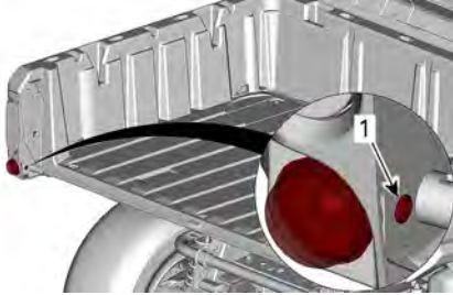
1. Borgschroef lens
