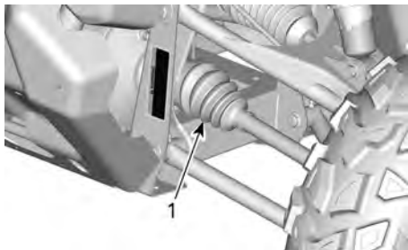
1. Balg binnenkant aandrijfswas
