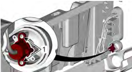
1. Borgschroeven
