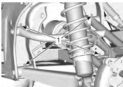
1. Smørenipler for bakke opphengssarm
