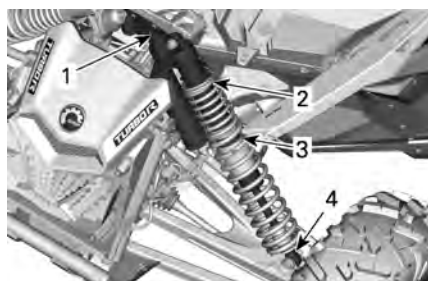
典型示例 - 带回弹阻尼 - 前悬架
