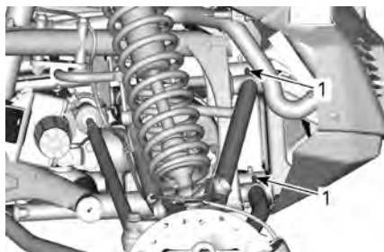
典型示例 - 前悬架
