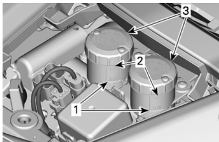
1. MIN (最低) 2. MAX 3. 主缸储液罐
